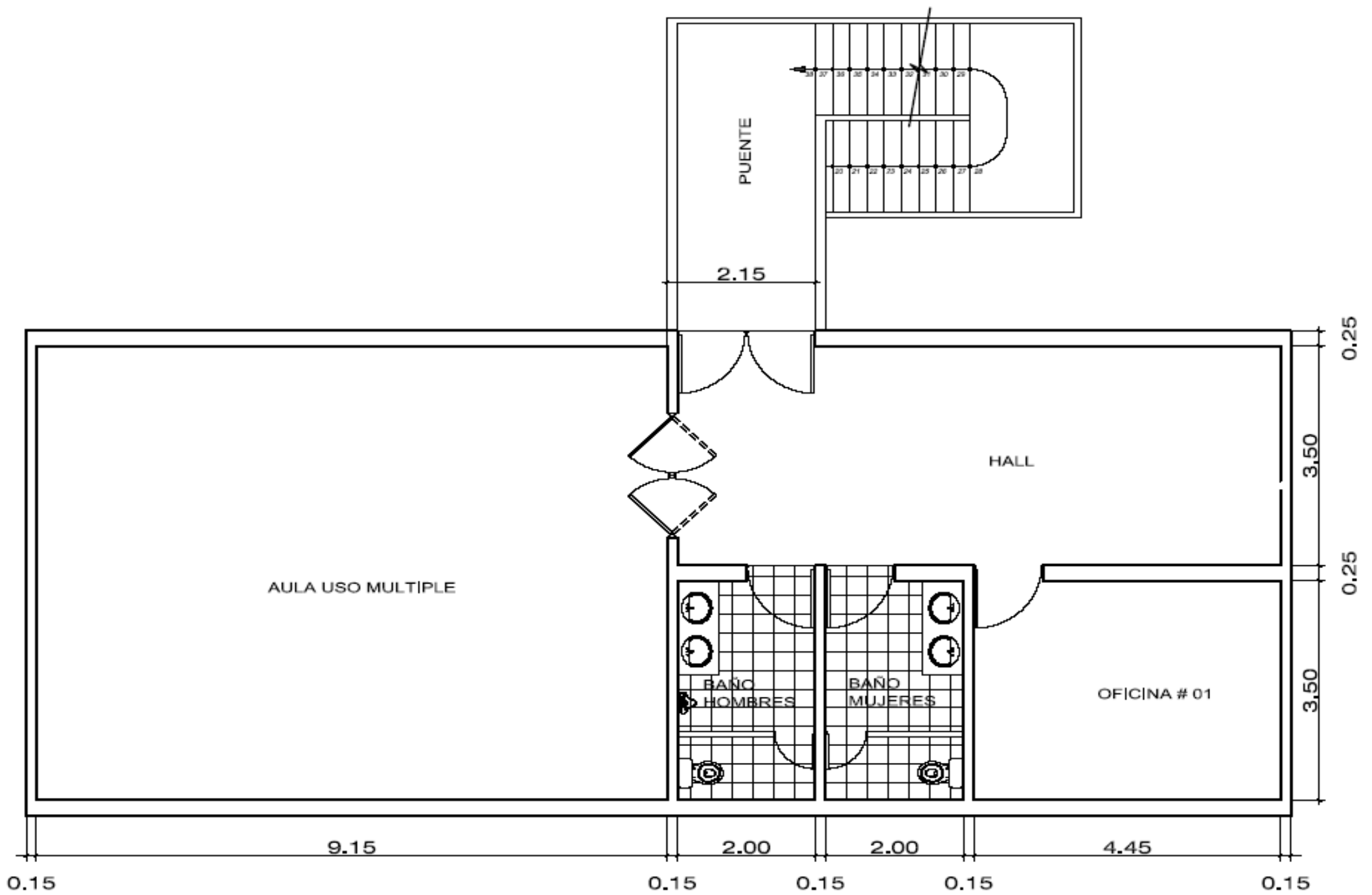
TERCER PISO - SALA DE REUNIONES
