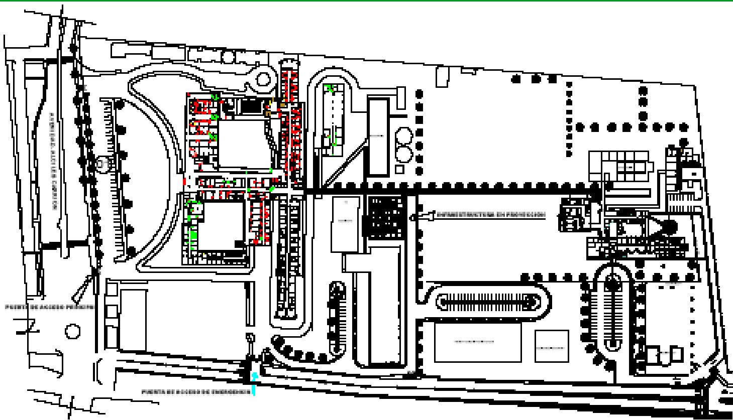
PLANIMETRIA EN GENERAL EBC-14002
